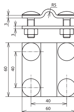
Maßbild
