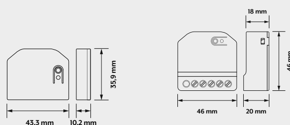
JUNG HOME Puck Binäreingang 2-fach, batterieversorgt
