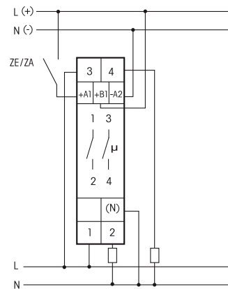
mit Kontaktschaltung im Nulldurchgang
